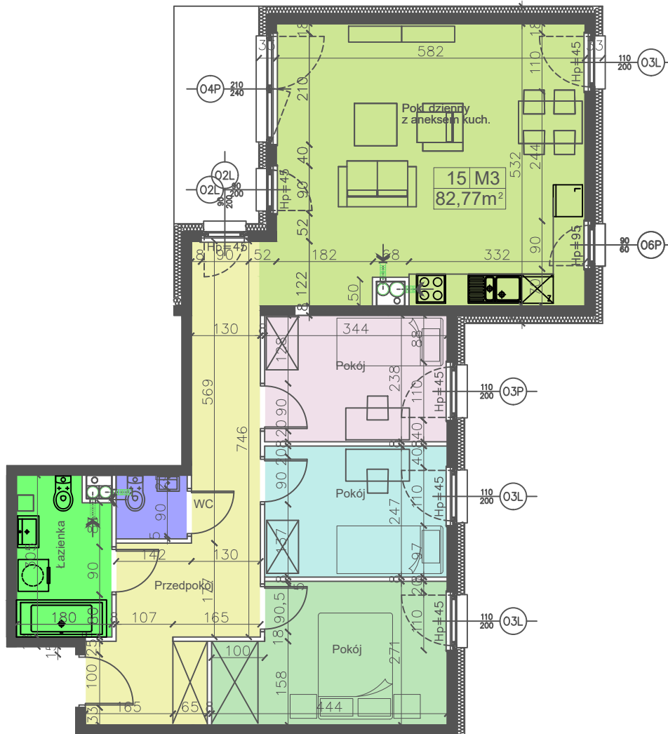
BUDYNEK D
